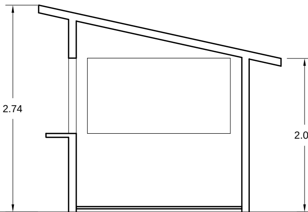
Secció
